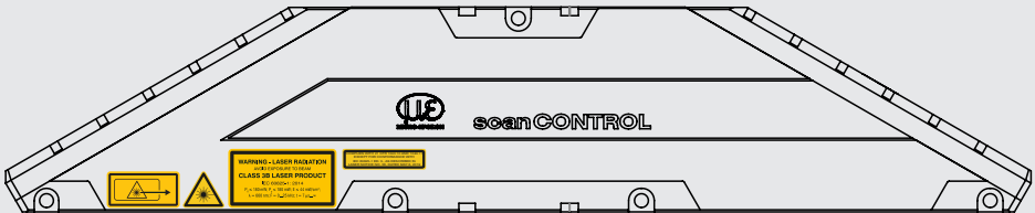
Fig. 10 Sensor LLT30xx-430, LLT30xx-600 with laser labels
