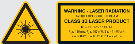
Fig. 9 Laser label and laser warning sign LLT30xx-430, LLT30xx-600
